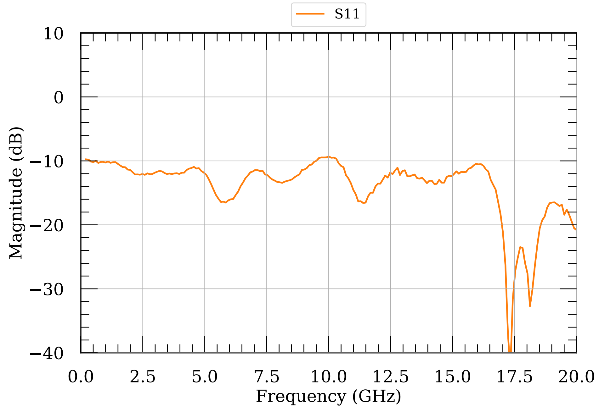
LNA S-params module013v2
